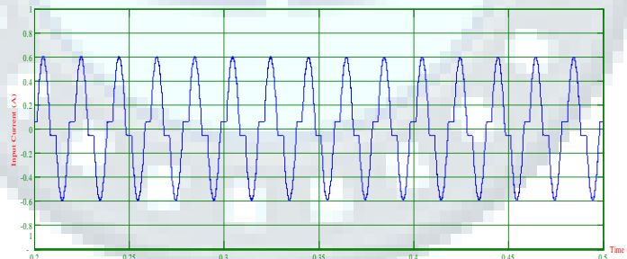
Fig. 13. Input current i_g
