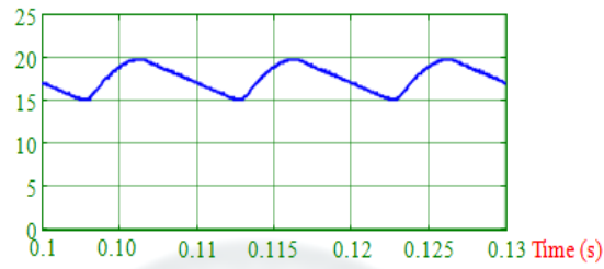
Fig. 15. Output voltage V_o
